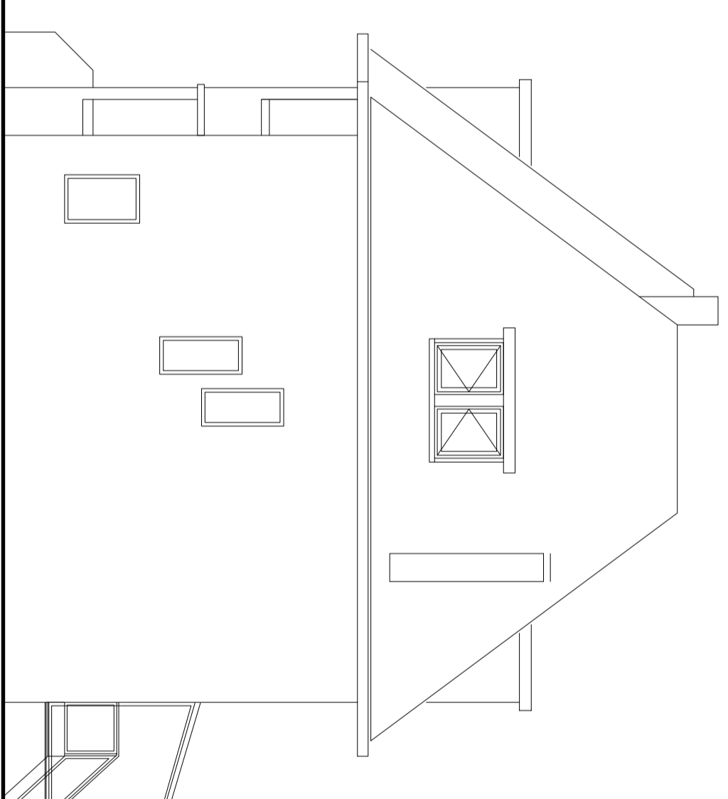
rechter zijgevel bestaand
