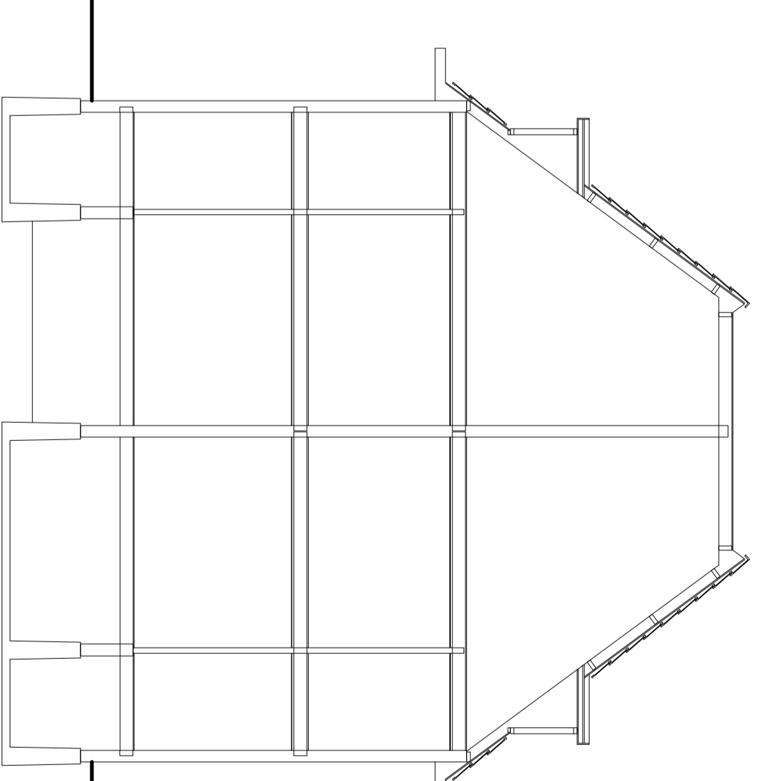
dwarsdoorsnede bestaand
