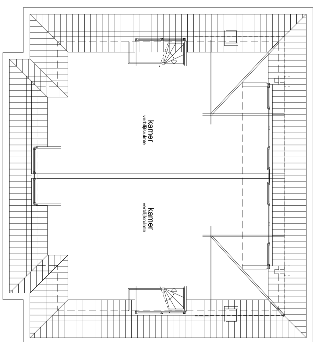
zolder bestaand
