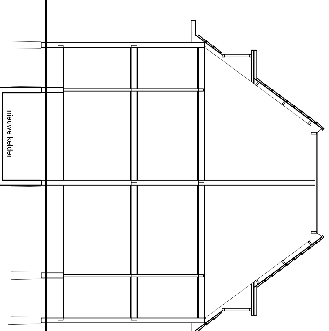
dwarsdoorsnede nieuw
